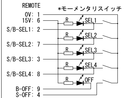
図5: MONO MODE SW接続例2 (1ボタン順次+OFF)
