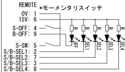
図3: ST MODE SW接続例3 (2ボタン選択)
