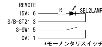
図2: ST MODE SW接続例2 (押す度反転)
