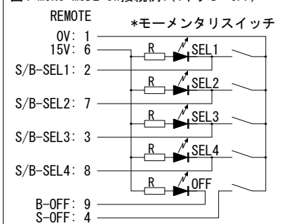
図5: MONO MODE SW接続例2(1ボタン順次+OFF)
