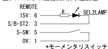
図2: ST MODE SW接続例2(押し度反転)
