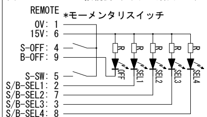
図3: ST MODE SW接続例3(2ボタン選択)
