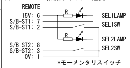
図3: ST MODE SW接続例3(2ボタン選択)
