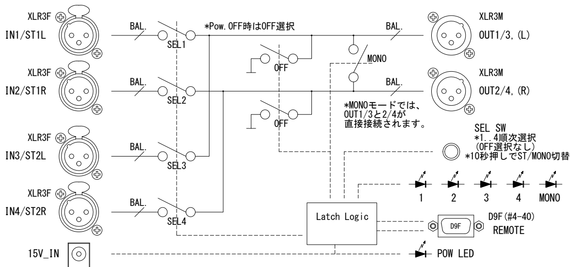
図4: MONO MODE SW接続例1(4ボタン+OFF)
